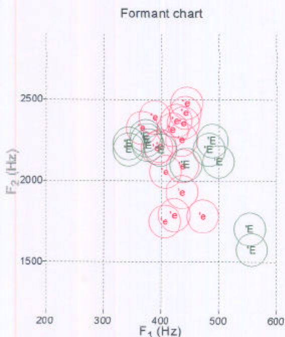
Figure 3 : [e] (en rouge) et [ɛ] (en vert) toniques chez LF
