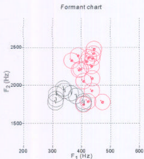
Figure 1 : [i] (en noir) et [e] (en rouge) toniques chez LF
