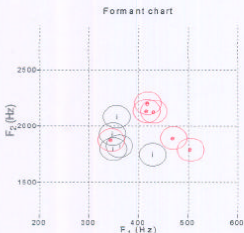
Figure 2 : [i] (en noir) et [e] (en rouge) atones chez LF
